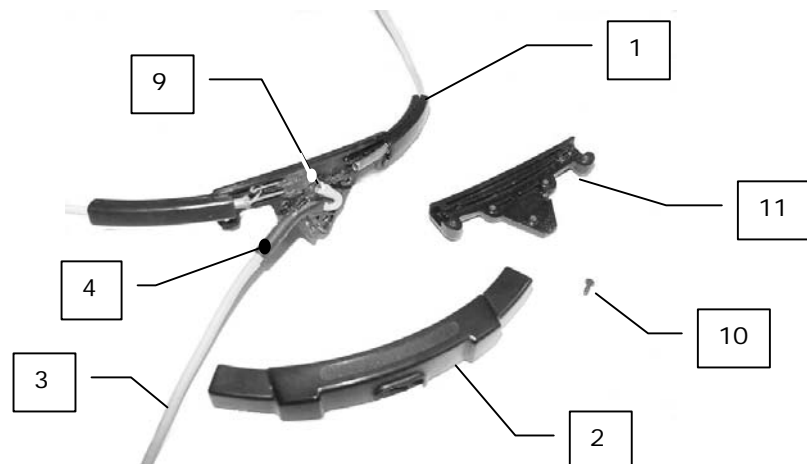
Connection piece with cable / Verbindungsstück mit Kabel
